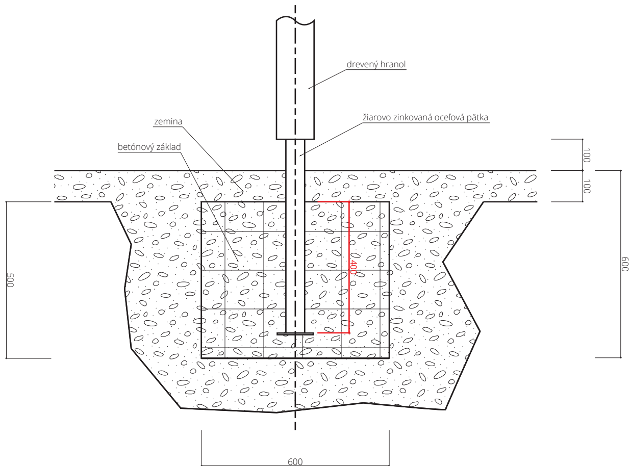
Detail ukotvenia
